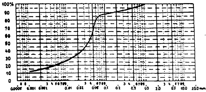
VII. tábla Tata-Porhanyóbánya üledékrétegeinek szemcseösszetéti burkoló görbéi
